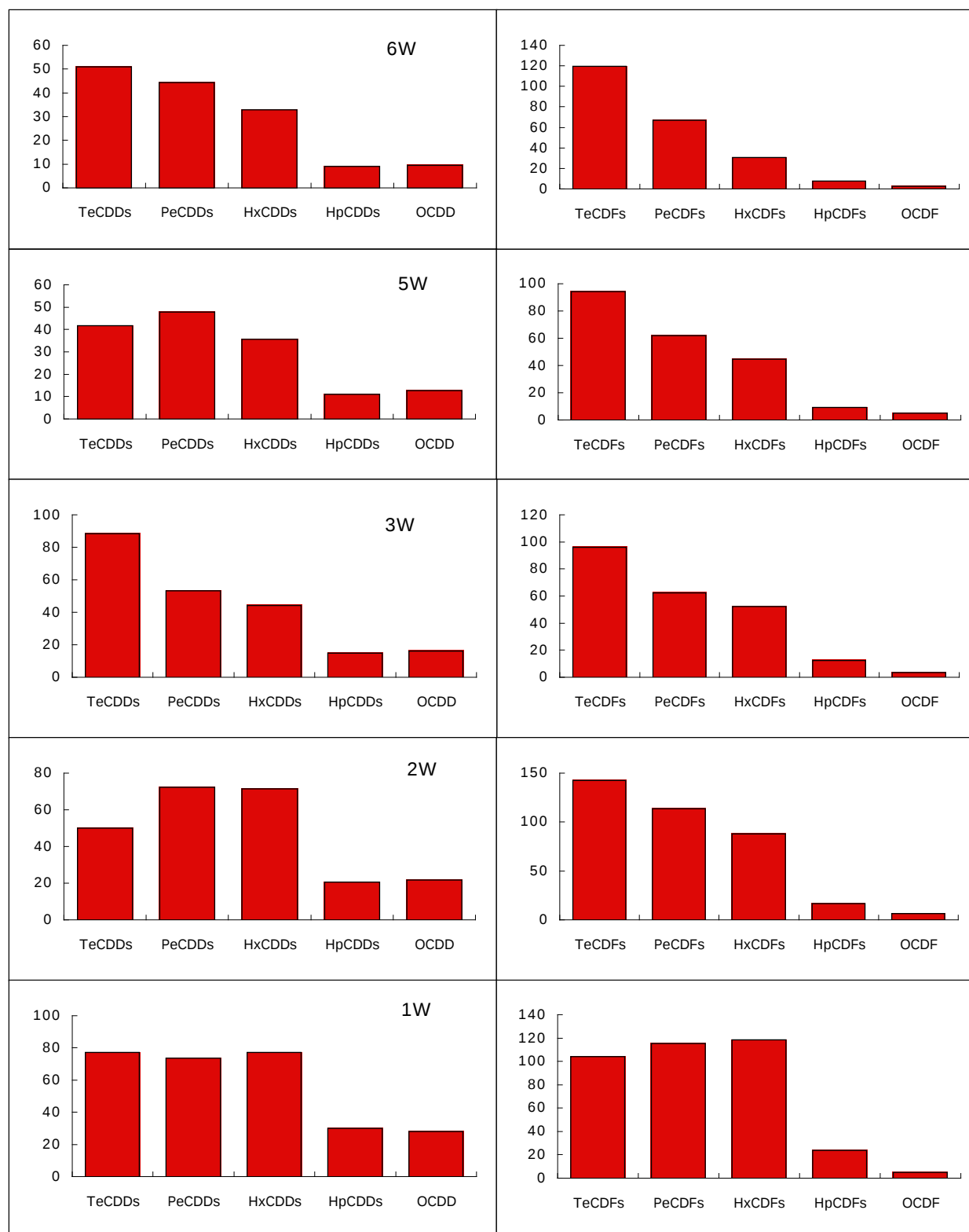
図3 クスノキに蓄積されたダイオキシン類の同族体分布 (1995.3.19-3.26)
